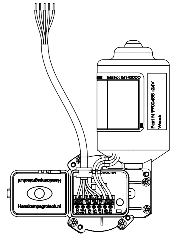
011-021-000 SolidState 5 motor
